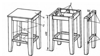
1 — передняя нога, 2 — сиденье, 3 — задняя нога, 4 — боковая нога, 5 — горизонтальная опора, 6 — подпятник.
